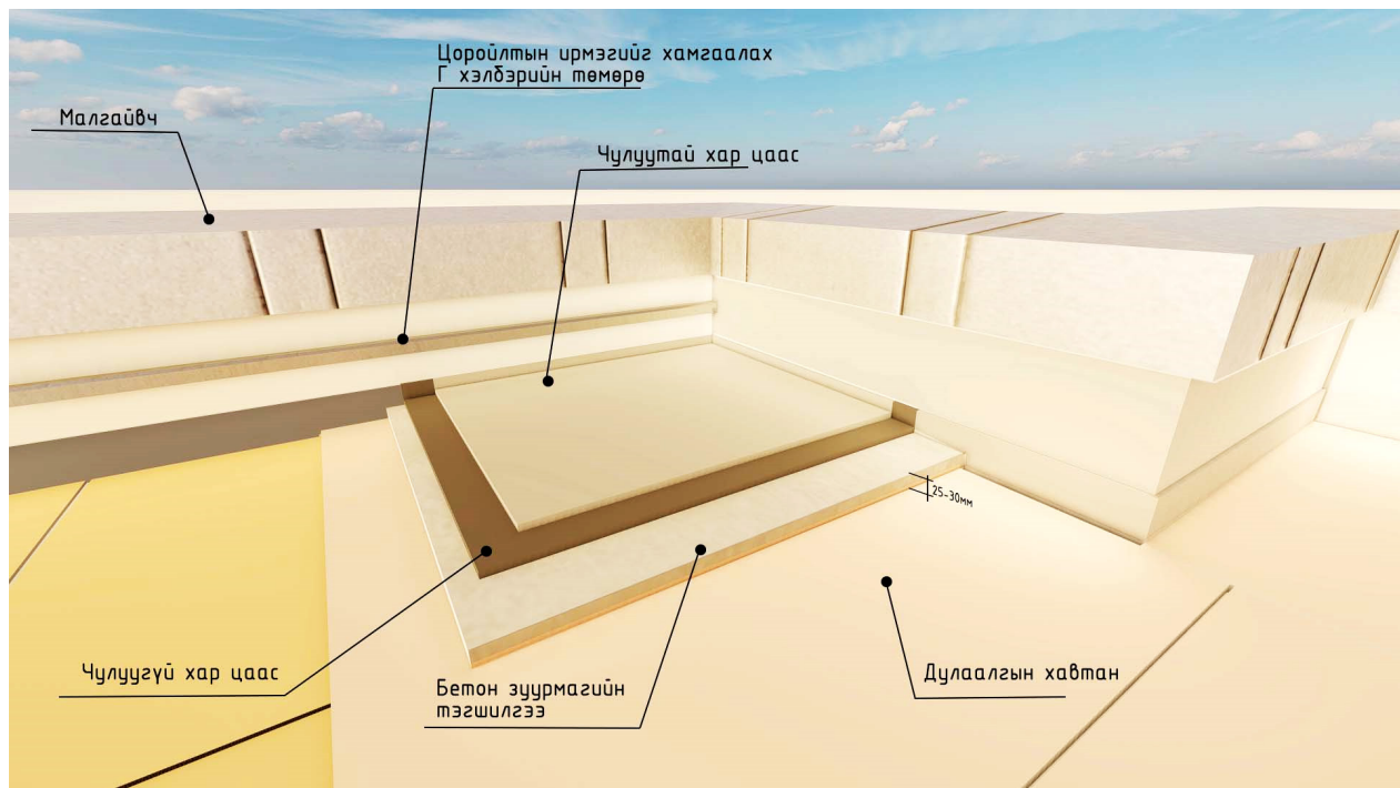
Зураг 4. Цоройлтын ирмэг болон малгайвч
