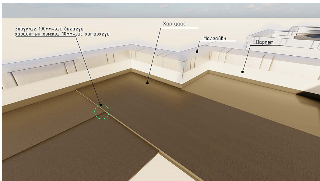
Зураг 2. Зөрүүлгийн хэмжээ (жишээ зураг)
