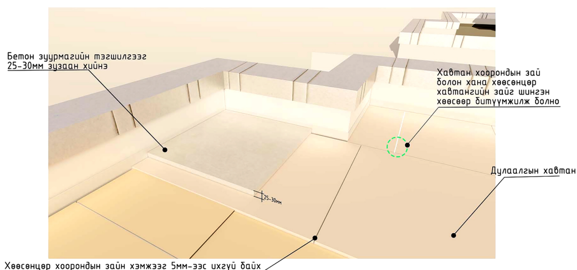
Зураг 5. Бетон зуурмагийн тэгшилгээ (жишээ зураг)
