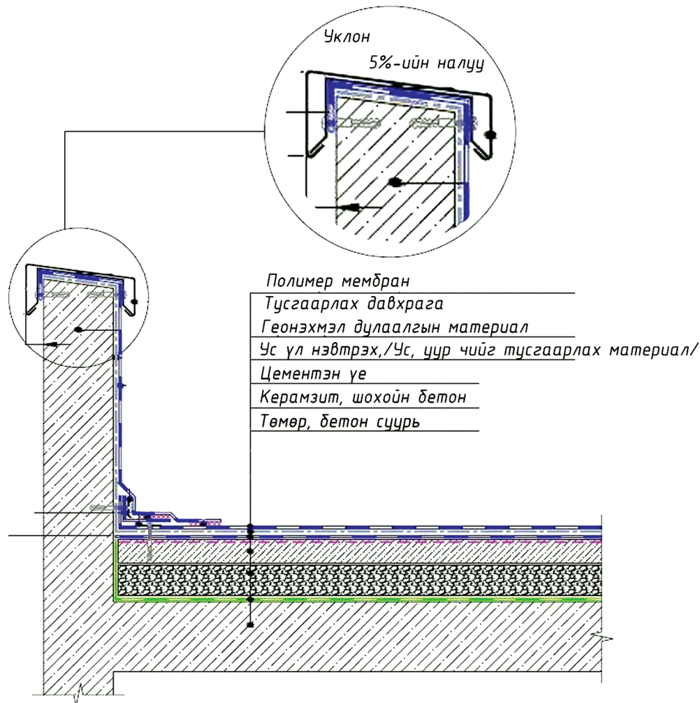
Зураг 3. Парпетны малгайвчны налуу (жишээ зураг)
